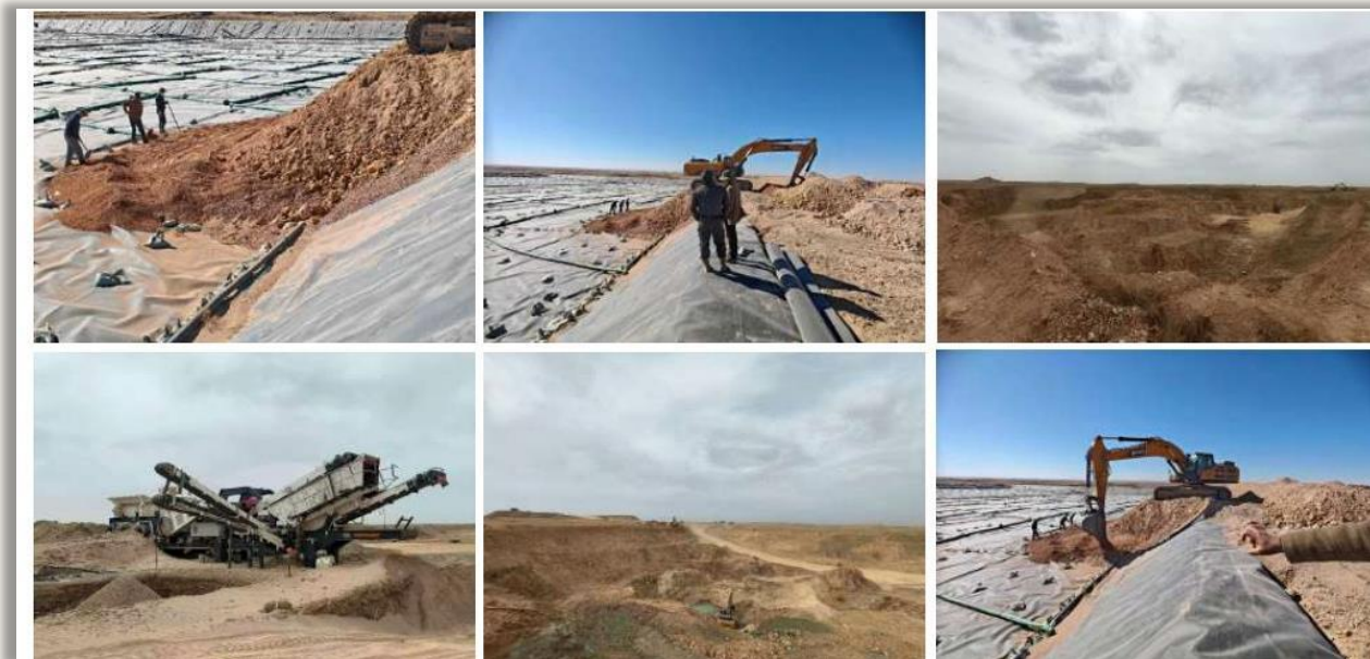
Хөрс хуулалт, овоолго болон нуруулдан уусгах талбайн ажлын явц.
